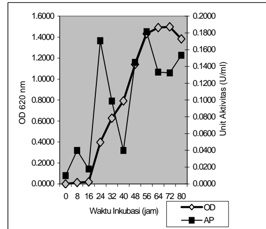
Gambar 2. Aktivitas Protease (AP) dalam media air rendaman kedelai dengan pH tidak terkontrol pada berbagai fase pertumbuhan mikroba (OD)
