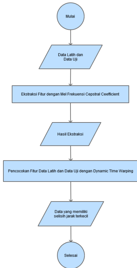
Gambar 6. Diagram Alir Sistem
