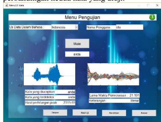
Gambar 12. Kata ‘Anda’ yang dikenali
