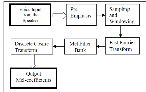
Gambar 2. Blok diagram untuk memperoleh MFC koefisien [7]
