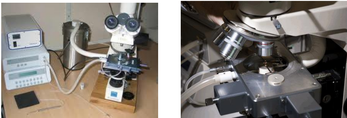
Gambar 2. Perangkat pengamatan inklusi fluida pada saat pengukuran T_h dan T_m .
