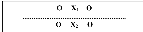
Gambar 1 Desain Penelitian
